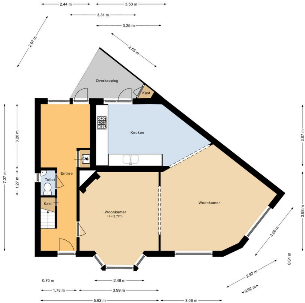
Begane grond Weteringkade 30 Noordwijk
